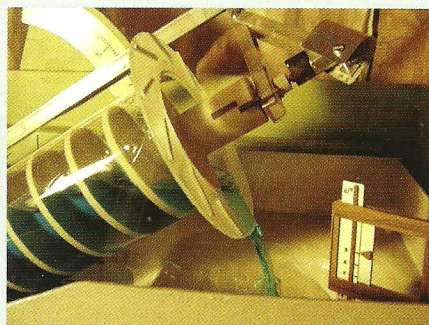
Maquette d'étude de la vis d'Archimède
