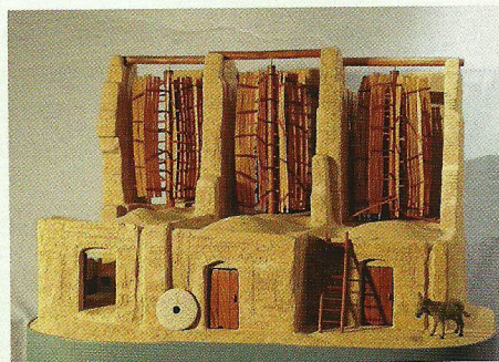
Moulins à vent céréalier, à axe vertical (IRAN)
